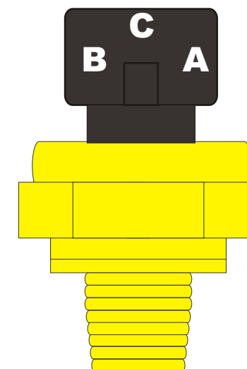
HALTECH 10 BAR PRESSURE SENSOR
